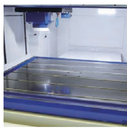
吸着+T溝兼用テーブル
